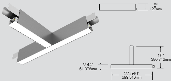
Tee
